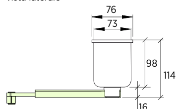
Motoriduttore e leva vista laterale
