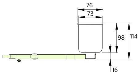
Motoriduttore e leva Vista laterale
