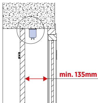
Sezione trasversale
