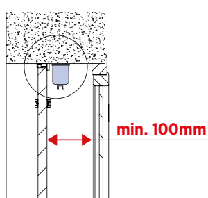
Sezione trasversale
