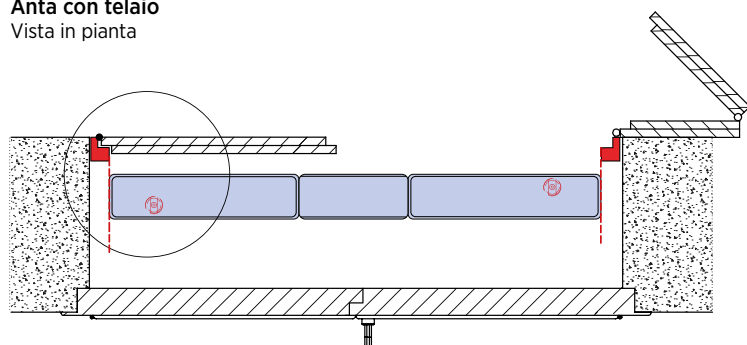
Anta con telaio
