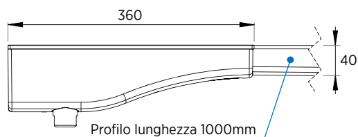
Vista frontale
