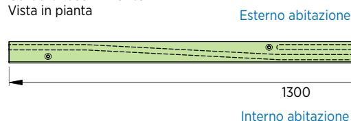
Guida di scorrimento Vista in pianta
