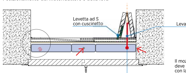
Posizionamento del motoriduttore e della leva
