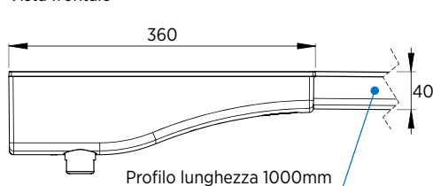
Vista frontale
