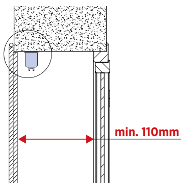
Sezione trasversale
