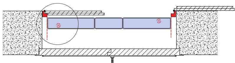
Vista in pianta
