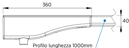
Vista frontale
