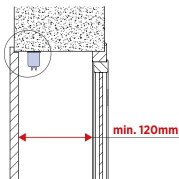
Sezione trasversale
