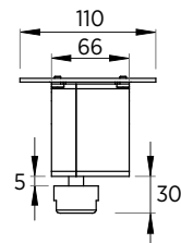
Motoriduttore con staffa Vista laterale
