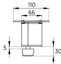
Motoriduttore con staffa Vista laterale
