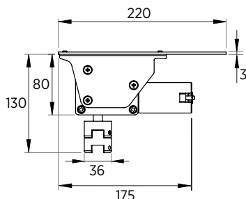
Guida di scorrimento Vista in pianta
