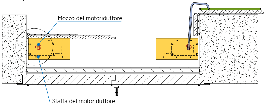
Posizione della staffa del motoriduttore Vista in pianta
