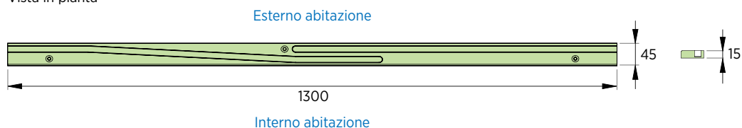
Guida di scorrimento Vista in pianta
