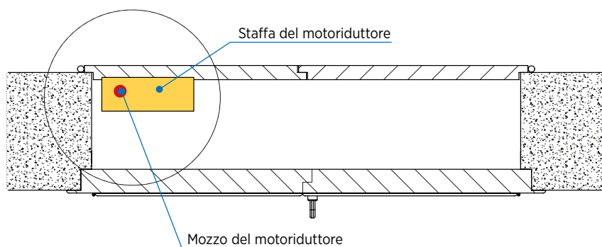
Posizione della staffa del motoriduttore Vista in pianta
