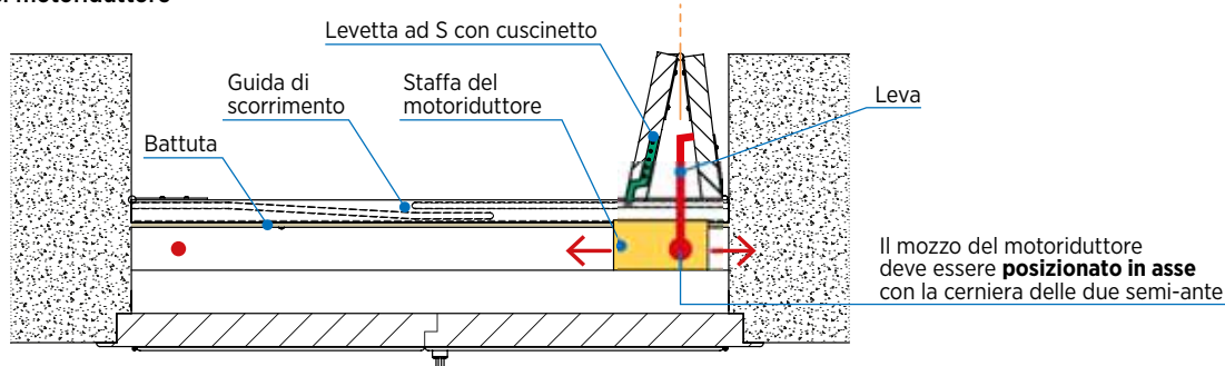
Posizione della staffa del motoriduttore Vista in pianta
