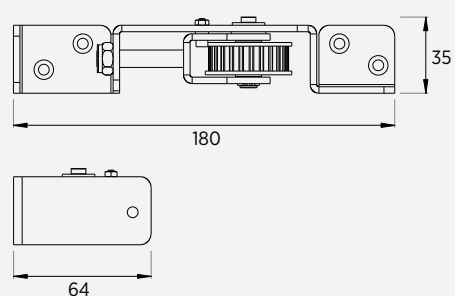
puleggia condotta
