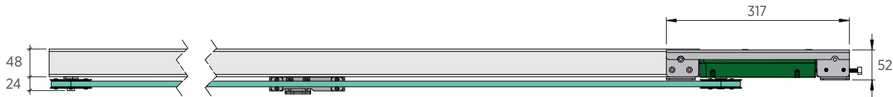
vista frontale
