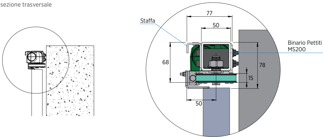
sezione trasversale
