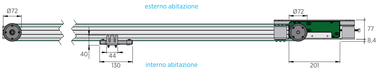
vista inferiore
